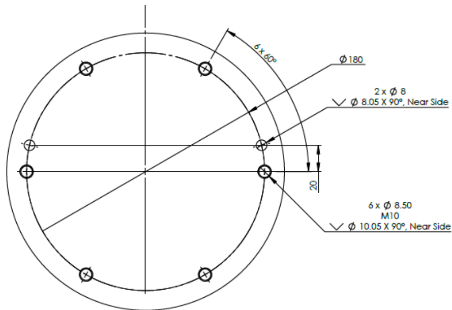
1.1: 機器人底座的底部視圖
